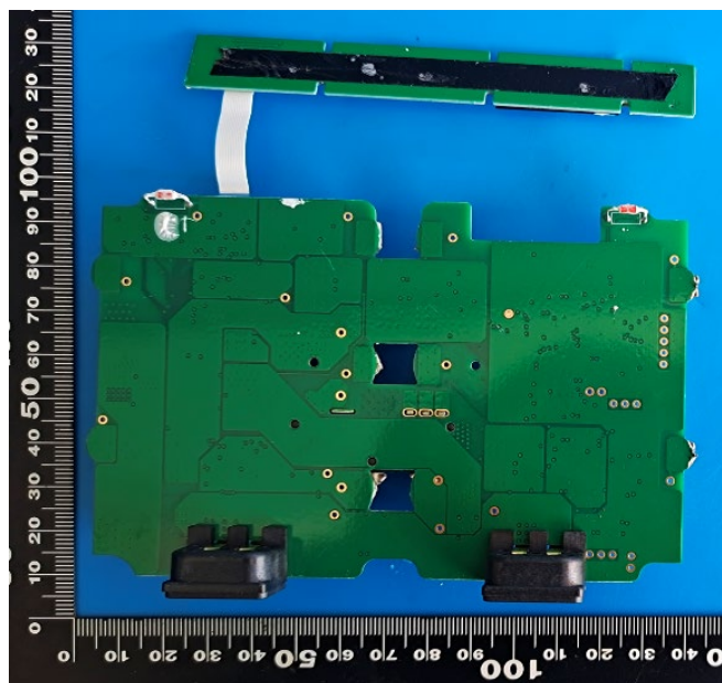
Fig. 6 – Back view of PCM 表6 – PCM 反面视图
