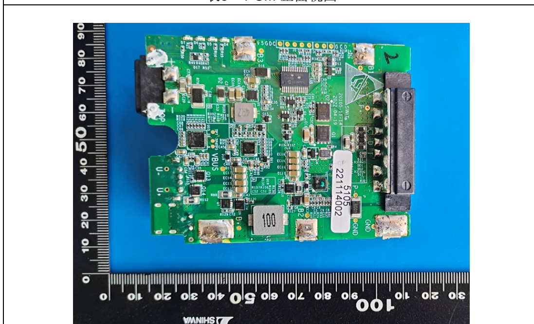
Fig. 5 – Front view of PCM 表5 – PCM 正面视图
