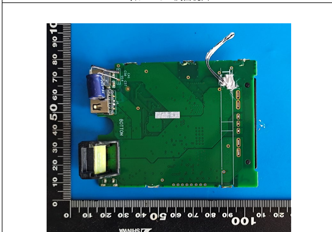
Fig. 6 – Back view of PCM 表6 – PCM 反面视图
