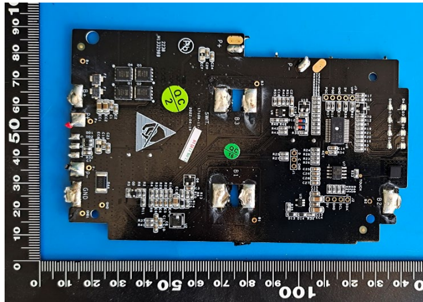
Fig. 5 – Front view of PCM 表5 – PCM 正面视图
