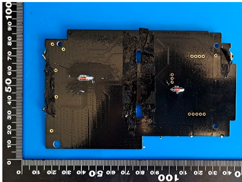
Fig. 6 – Back view of PCM 表6 – PCM 反面视图
